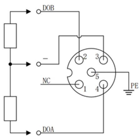
PNP输出
