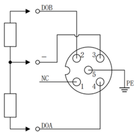
PNP输出
